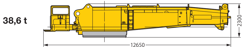
上部旋回体(クイックコネクション付)
