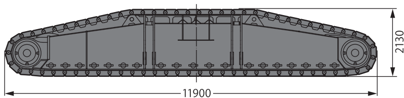
クローラシュー & ドライブギア
