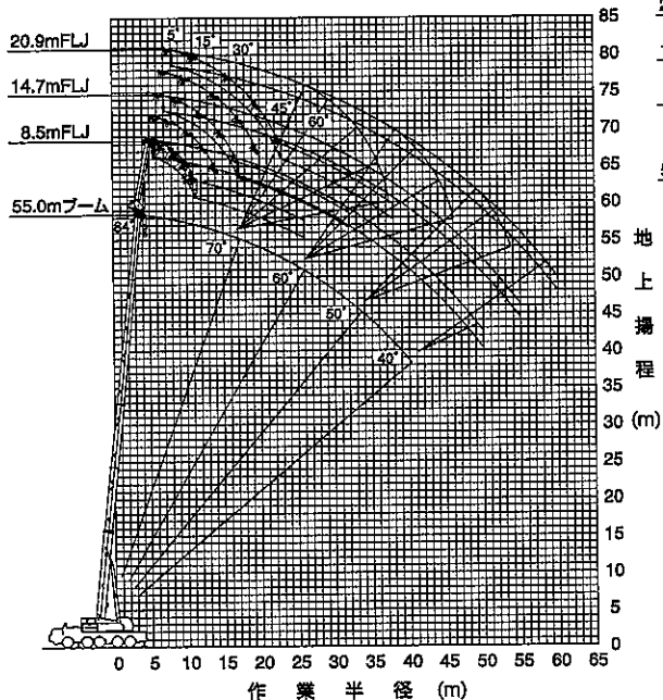
55.0mブーム+1.85m+フルオートラフティングジブ
