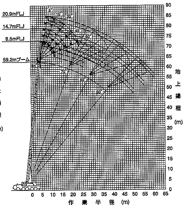
59.2mブーム+1.85m+フルオートラフティングジブ
