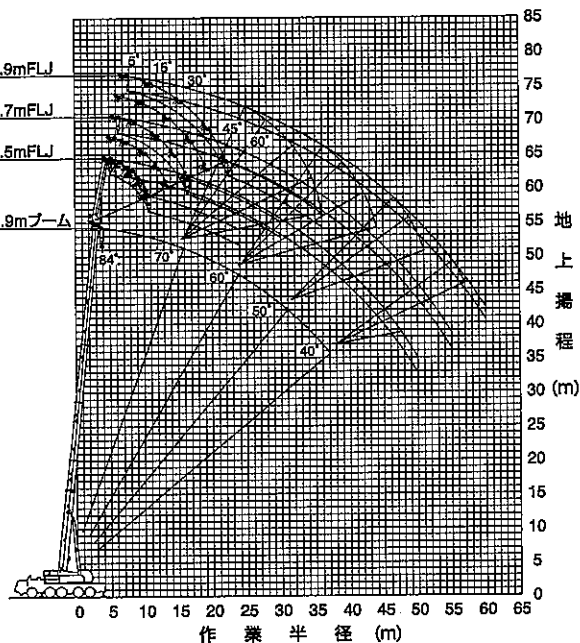
50.9mブーム+1.85m+フルオートラフティングジブ
