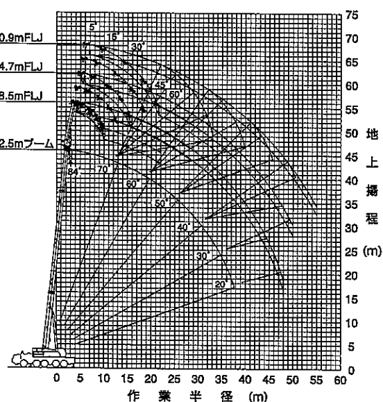
42.5mブーム+1.85m+フルオートラフィングジブ
