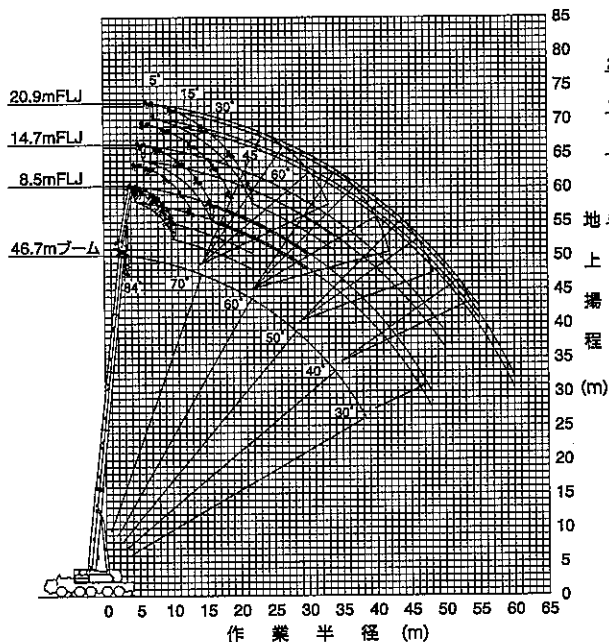
46.7mブーム+1.85m+フルオートラフティングジブ
