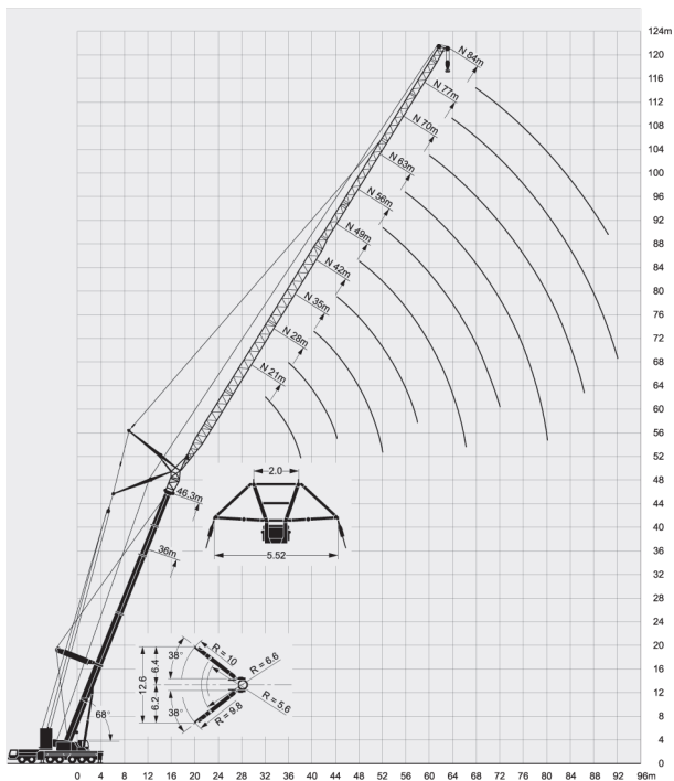
メインブーム 68°
