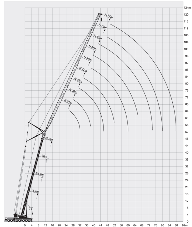
メインブーム75°
