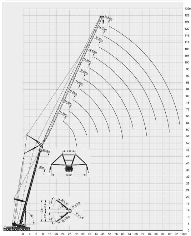
メインブーム 75°
