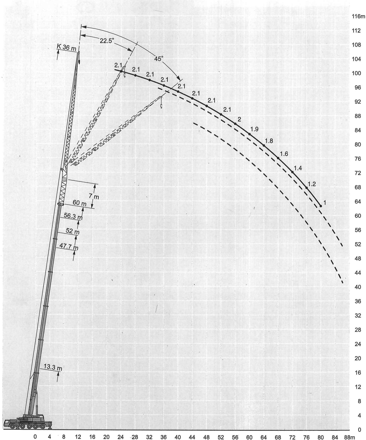
油圧チルトジブ (ブームエクステンション付) 定格総荷重表
