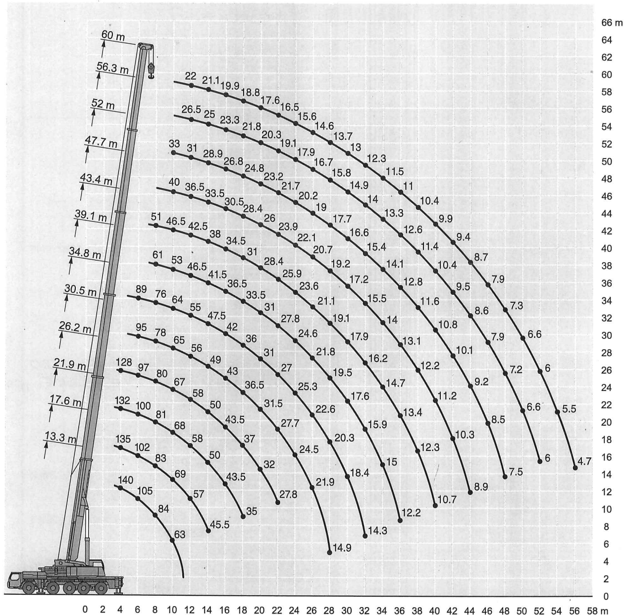
メインブーム定格総荷重表
