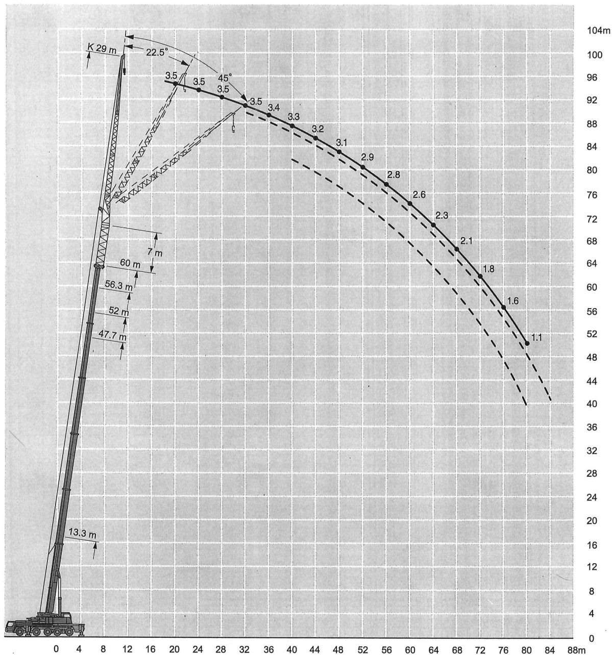
油圧チルトジブ (ブームエクステンション付) 定格総荷重表
